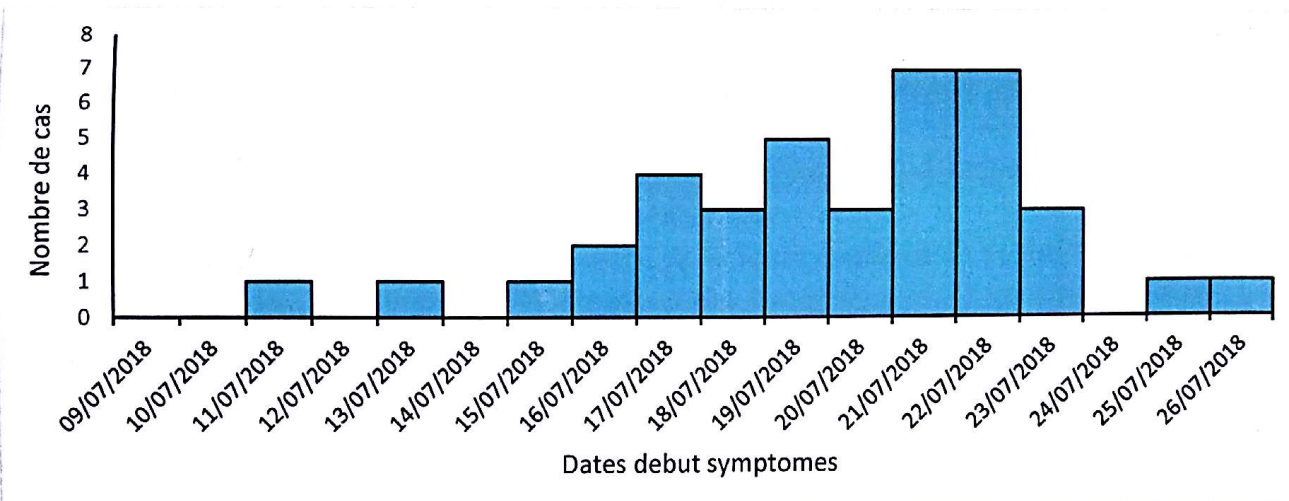
Fig 1 : Courbe épidémique des cas de choléra dans la Région du Centre, 26 juillet 2018
